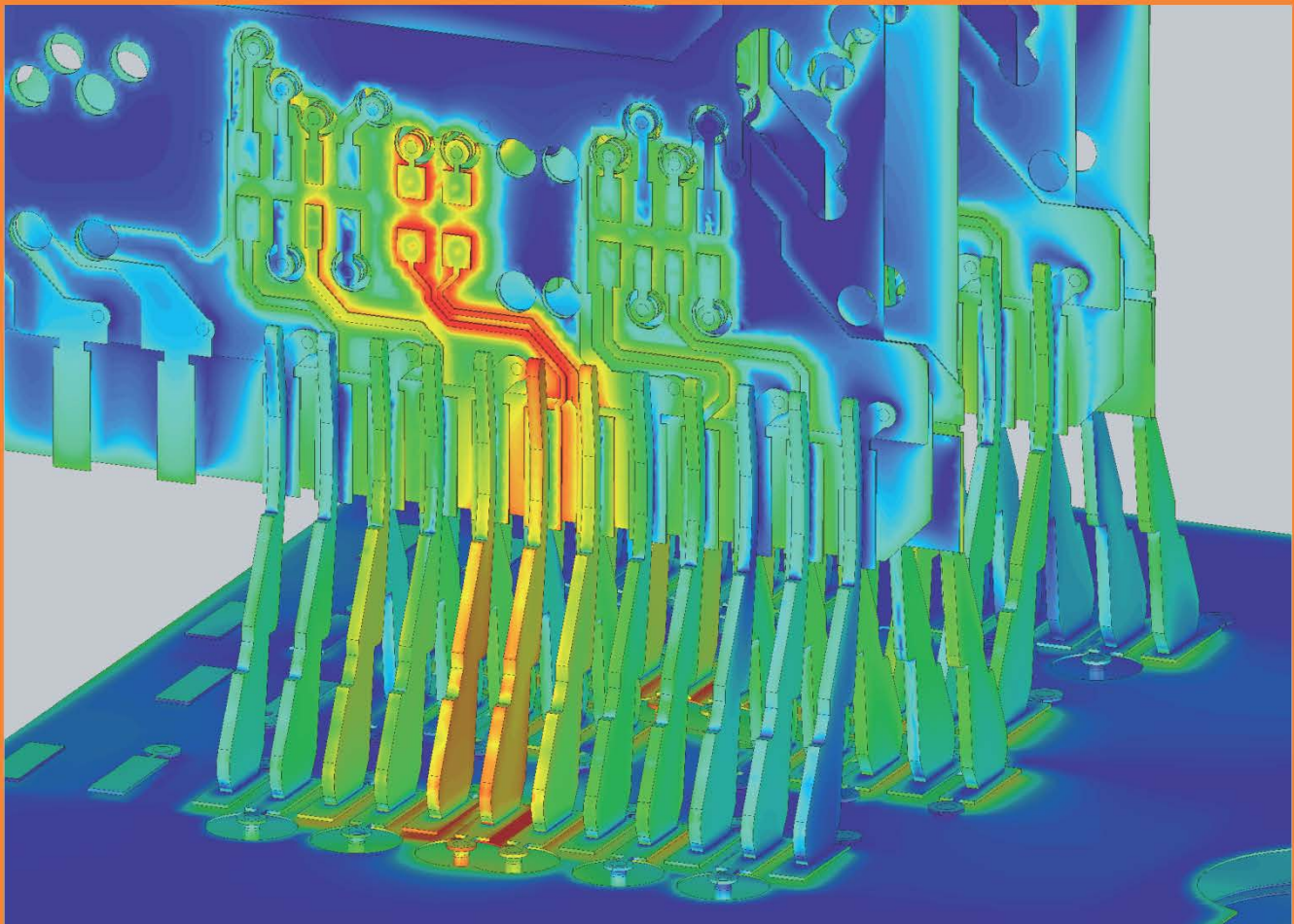
Результат моделирования электрического поля в канале модулей ОЗУ DDR4.
