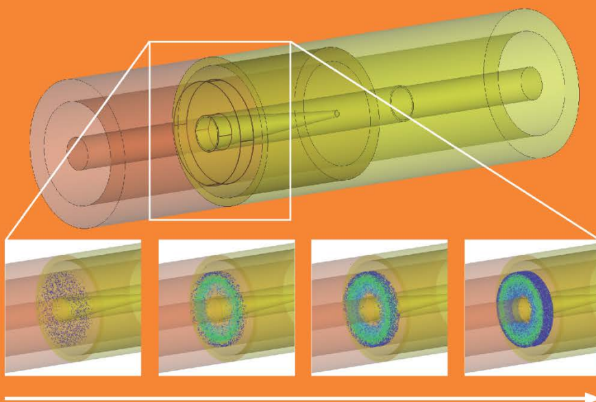
Моделирование каскада электронов, возникающего внутри коаксиального разьема. Наблюдаемый мультипакторный разряд может привести к разрушению устройства.
