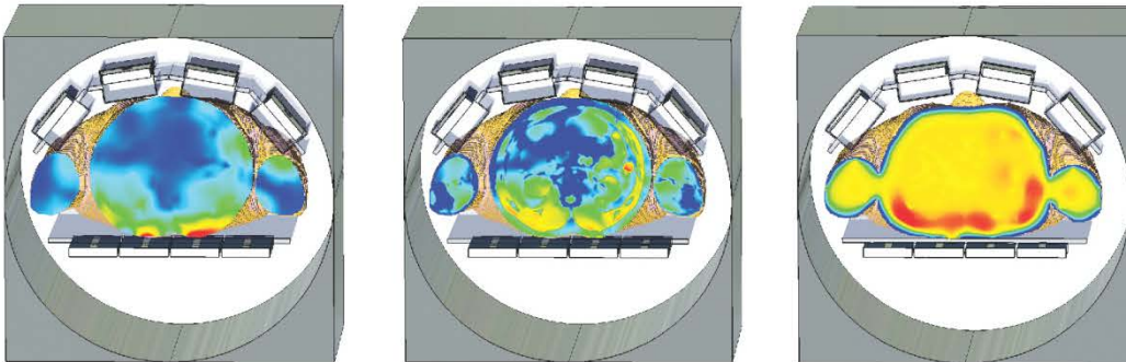
С помощью проекта магнитно-резонансного томографа 7 Tesla MRI, включающего 8 меандровых микрополосковых элементов и подробную воксельную модель тела человека были получены: распределение поля B_1^+ (слева), точка SAR (в центре) и распределение температуры внутри тела после 10 минут облучения (справа). Пример предоставлен институтом Erwin L. Hahn Institute for MRI, Эссен, Германия.
