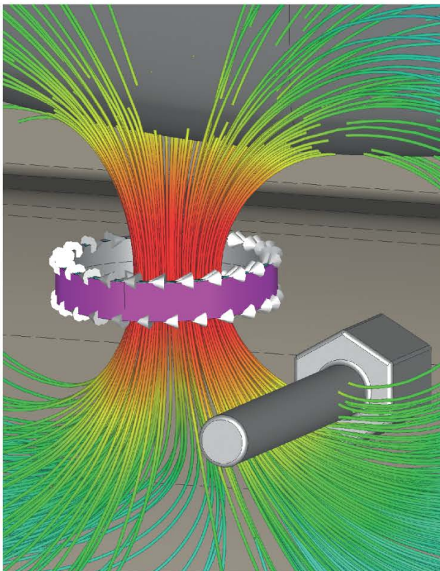
Линии магнитного поля вокруг катушки встраиваемого колесного датчика показывают взаимодействие ее с колесной парой.
