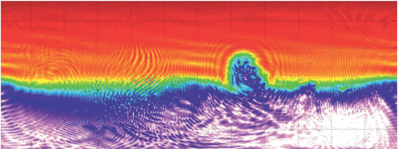
Моделирование характеристик слабонаправленной антенны с помощью MLFMM вычислителя на основе интегральных уравнений. Хорошо заметна область тени от расположенной рядом направленной антенны.
