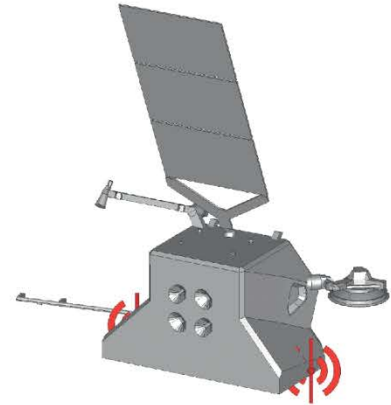
Пример моделирования размещения антенн на спутнике VeriColombo Mercury Planetary Orbiter. Слабонаправленные антенны представлены в виде источников поля.
