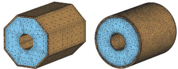
Различные способы построения сетки разбиения для коаксиального волновода: традиционный (слева) и адаптивный True Geometry Adaptation (справа).
