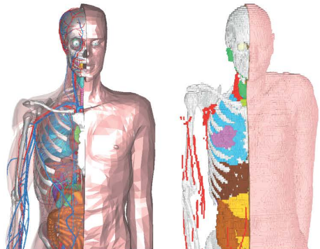
Для выполнения EM моделирования CST предлагает пользователям CAD-модели (слева) или воксельные модели (справа) человеческого тела.
