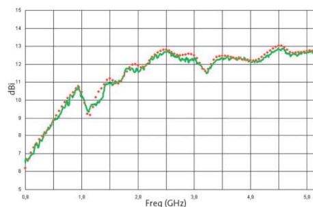
Прекрасное согласование в широком диапазоне частот измеренных и рассчитанных характеристик двухгребневой рупорной антенны Сатимо.
