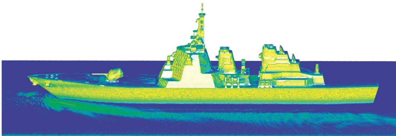
Распределение токов на металлической поверхности корабля длиной 155 метров и облучаемого плоской волной сигнала с частотой 400 МГц. При моделировании учитывалась относительная диэлектрическая проницаемость соленой воды (81) и ее удельная проводимость (0.01 См/м)
