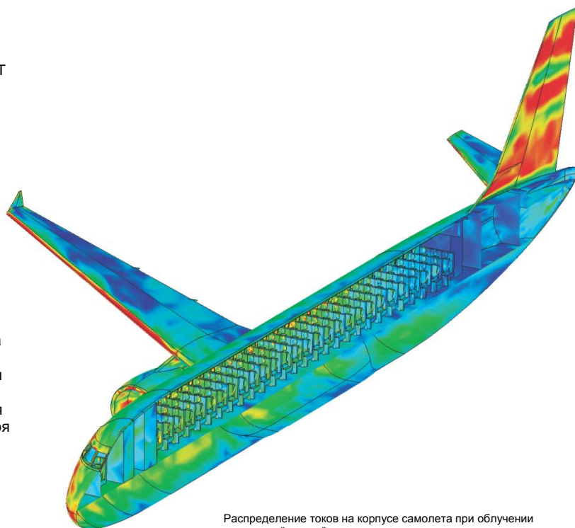
Распределение токов на корпусе самолета при облучении его плоской волной.
