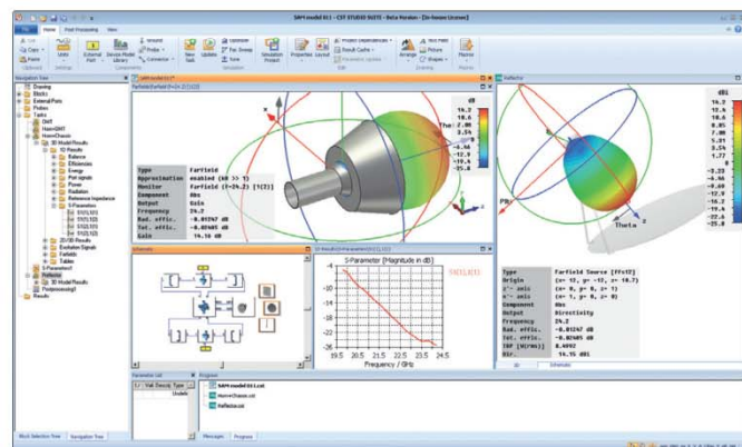
Пример технологии SAM: несколько проектов отдельных частей устройства объединяются в одном проекте и моделируются совместно (селектор поляризации, рупорная антенна и рефлектор).
