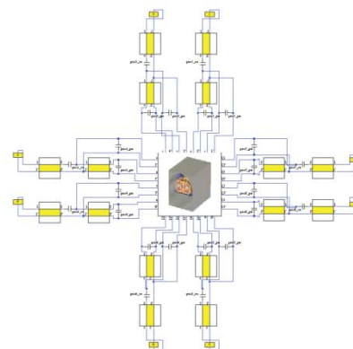
Схема для настройки и оптимизации MRI системы
