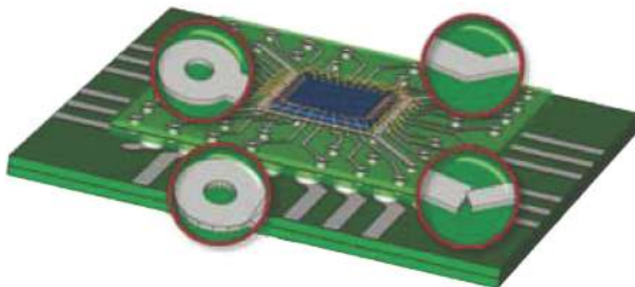
После импорта трехмерной структуры на ней подсвечиваются автоматически выявленные и исправленные ошибки CST MWS данных (увеличено).
