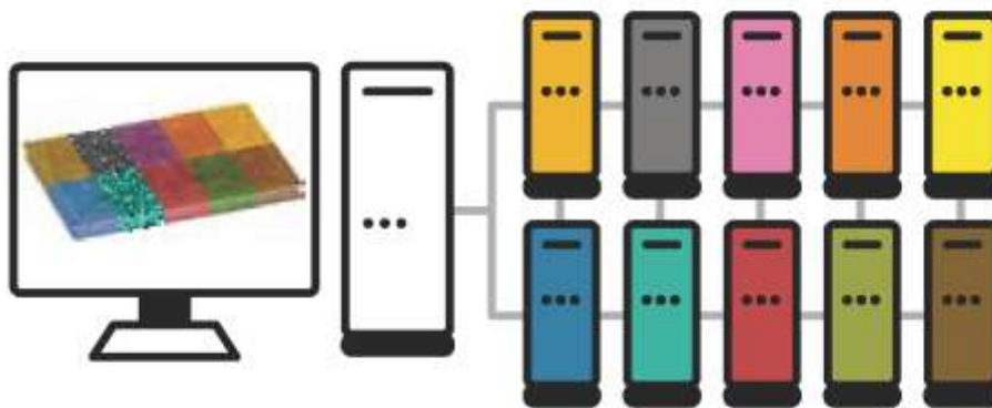
Пример использования декомпозиции сложного проекта. Интерфейс MPI распределяет отдельные части проекта для анализа на нескольких компьютерах в рамках сети.
