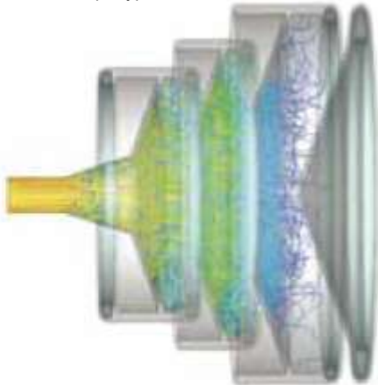
СВЧ коллектор с рекуперацией: электроны замедляются электростатическими полями и поглощаются металлическими стенками, моделируется вторичная электронная эмиссия. В результате анализа получают траектории элементарных частиц (слева), а также распределение тепла в конструкции (справа).
