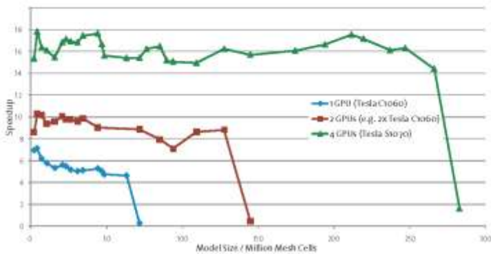
Прирост производительности вычислений при использовании разных графических процессоров (GPU) по сравнению с системой на базе двух процессоров Intel Xeon X5550.
