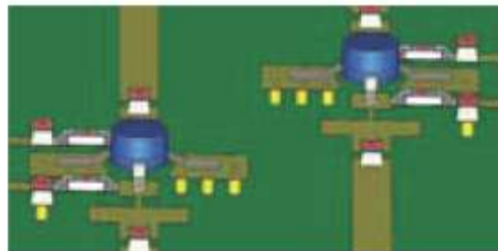
Широкополосный балансный усилитель мощности диапазона 3 – 5 ГГц промоделированный во временной области как схема с EM структурами.
