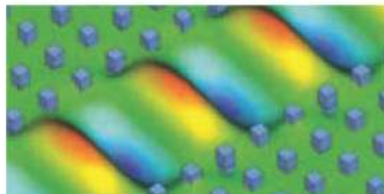
Линейный дефект волновода в фотонном кристалле.
