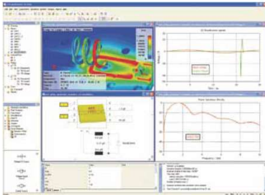
Сквозное моделирование проекта наносекундного генератора импульсов на уровне схемы и EM структуры. Сигнал с частотой 60 МГц преобразуется в сверхкороткий импульс, который подается на диод с накоплением заряда с ярко выраженной нелинейностью.
