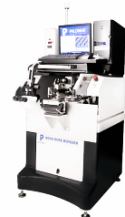
Автоматическая установка ультразвуковой микросварки Palomar 8000i
