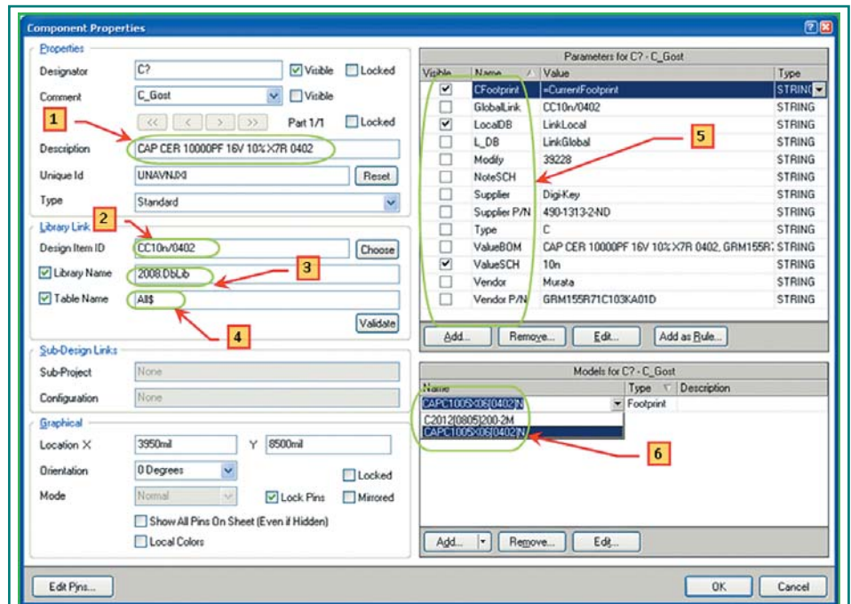
Рис. 8. Параметры компонента из Database Library
